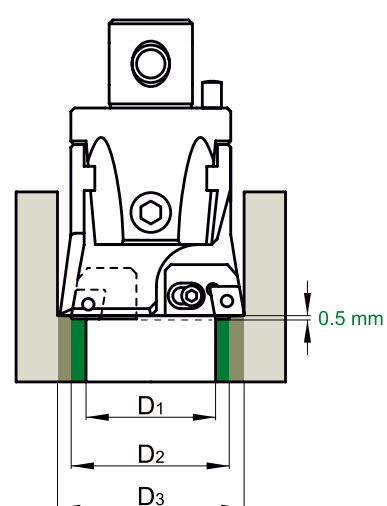
Alésage décalé
