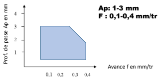
Diagramme d'utilisation du brise copeau ADF :
