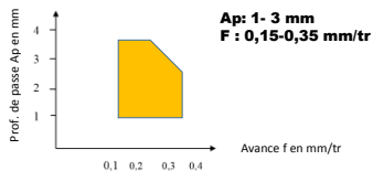
Diagramme d'utilisation du brise copeau SNR :
