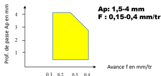
Diagramme d'utilisation du brise copeau EG :
